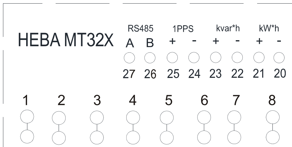
Схема подключения испытательных выходов счетчиков НЕВА МТ32Х (кроме исполнений НЕВА МТ32Х /5(10) А)
