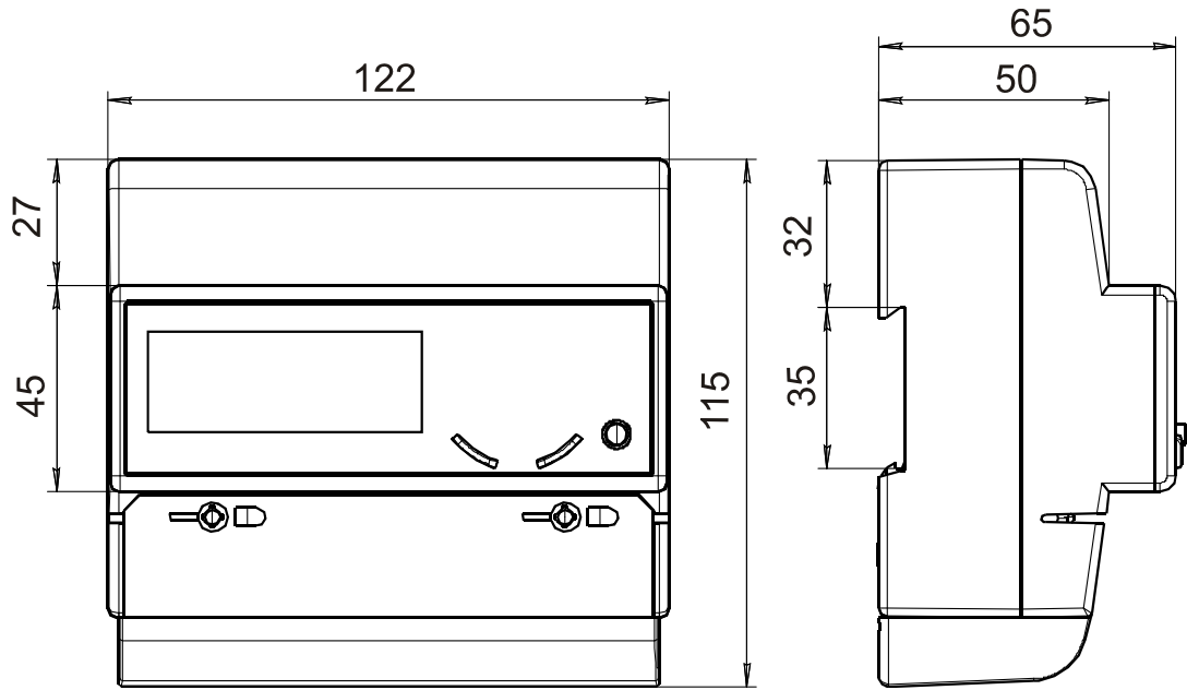
Внешний вид счетчиков НЕВА МТ32Х
