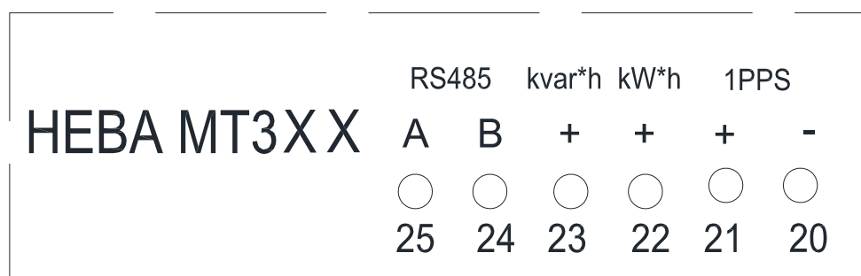
Схема подключения испытательных выходов счетчиков НЕВА МТ32Х /5(10) А и счетчиков НЕВА МТ31Х (кроме исполнений НЕВА МТ31Х XXXSR)
