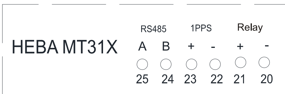
Схема подключения испытательных выходов счетчиков НЕВА МТ31Х XXXSR
