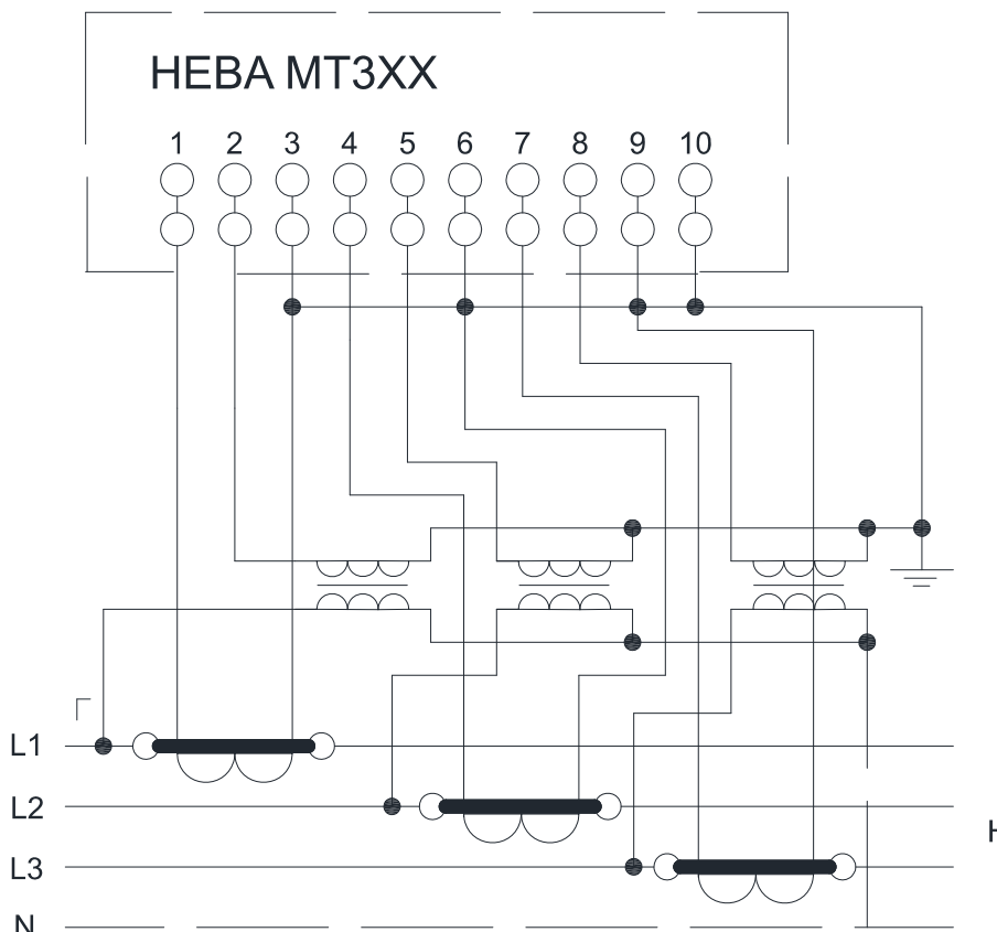
Схема включения счетчиков HEBA MT3XX через трансформаторы тока и трансформаторы напряжения в четырёхпроводную сеть
